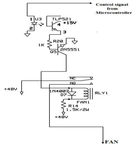
Fig. 6. Fan Driving Section
